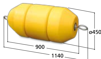
UB-110 Volym 110 liter Art. nr 30087 Vikt 14,0 kg
