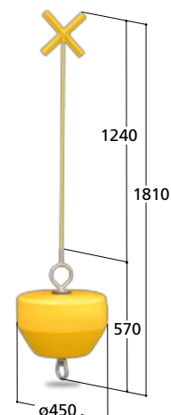
UMB-30 Markeringsboj Volym 30 liter Art. nr 30084 Vikt 8,0 kg
