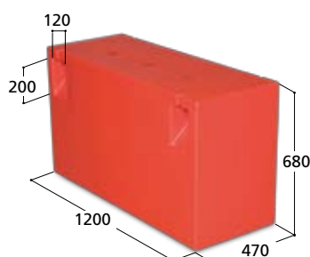
Volym 375 liter Art. nr 30125 Vikt 33,0 kg
