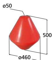
Volym 40 liter Art. nr 30032 Vikt 3,0 kg
