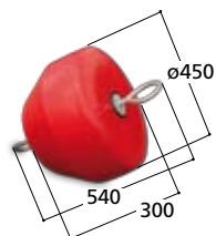
UB-30 Volym 30 liter Art. nr 30085 Vikt 6,0 kg
